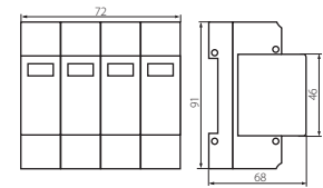
KSD-T2 275/160 3P+N
